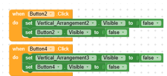
Рисунок 19 - Блоки для работы кнопок «Button2» и «Button4»
