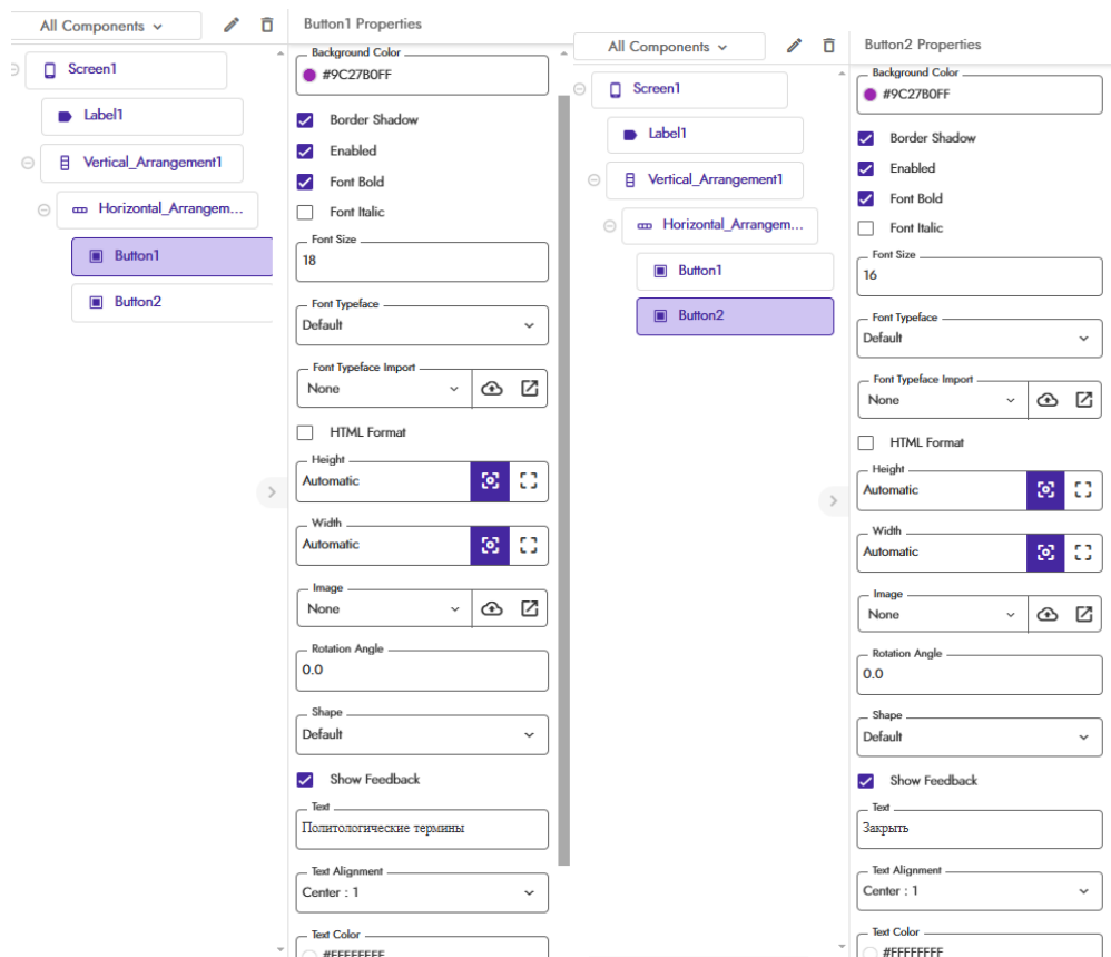
Рисунок 7 - Свойства компонентов «Button1» и «Button2»
