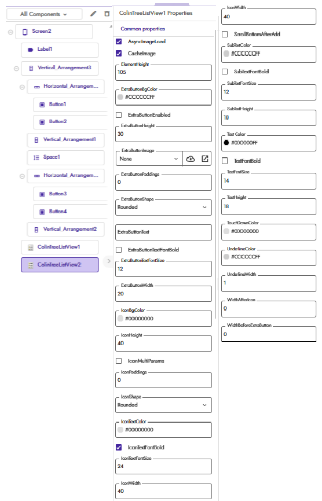
Рисунок 15 - Изменение свойства расширения «Colintreelistview2»
