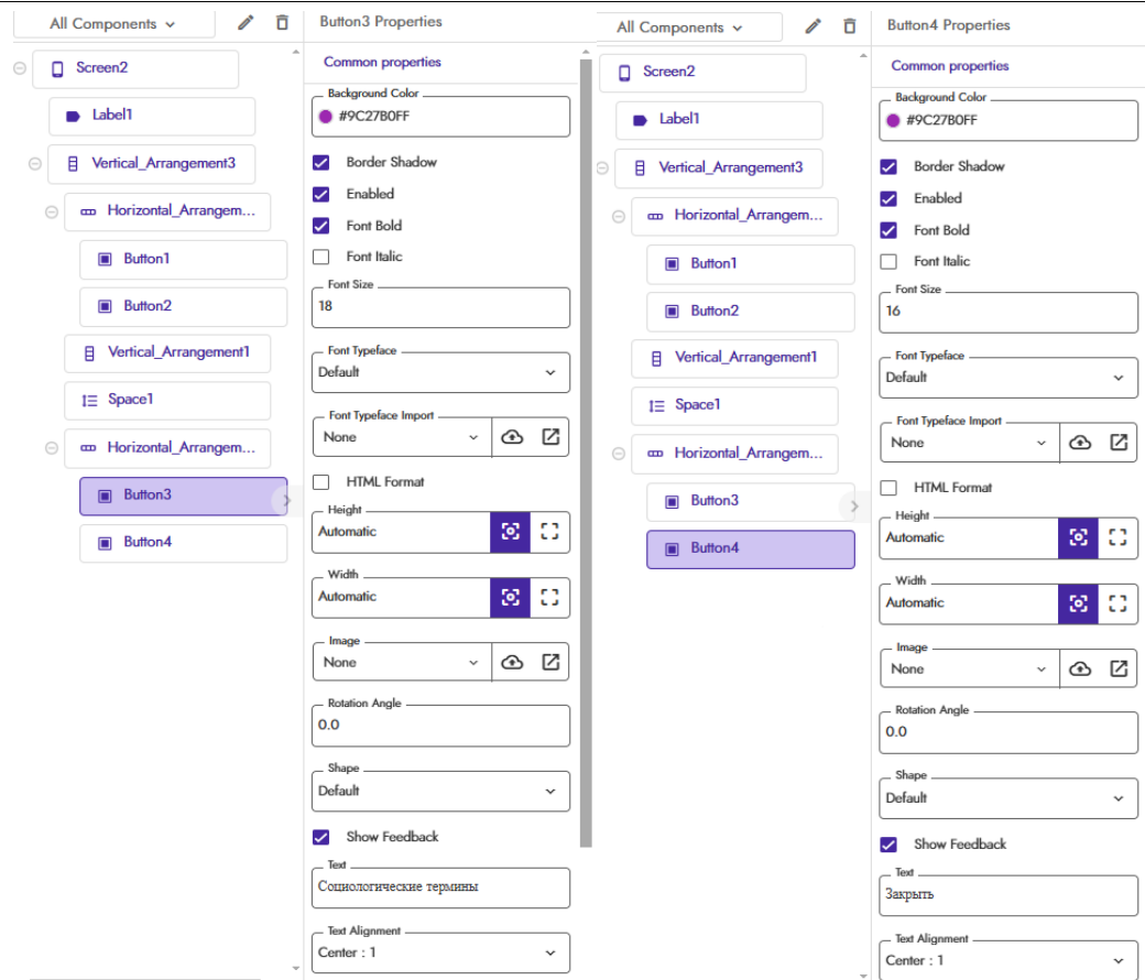
Рисунок 11 - Свойства компонентов «Button3» и «Button4»
