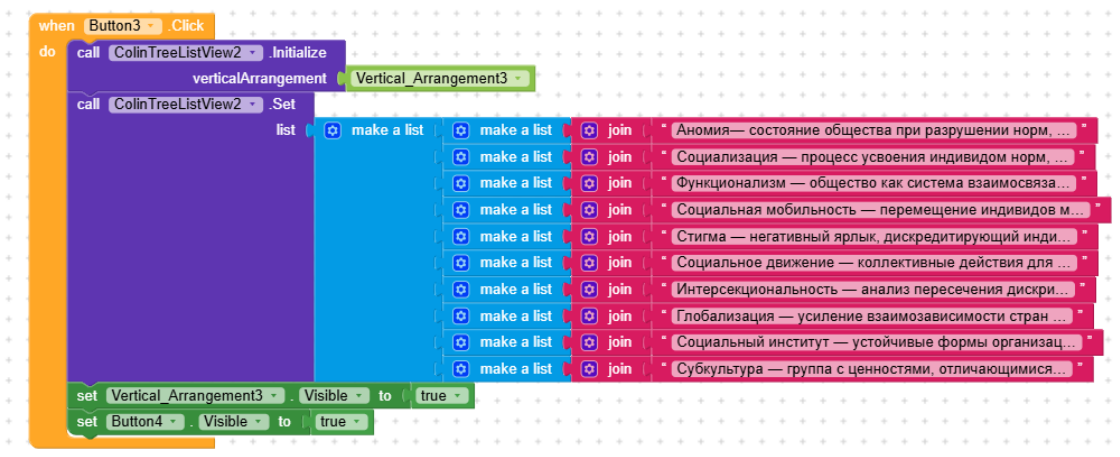
Рисунок 18 - Блок для работы кнопки «Button3»
