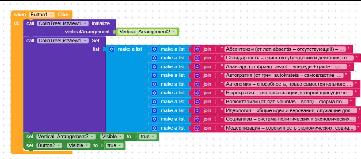
Рисунок 17 - Блок для работы кнопки «Button1»
